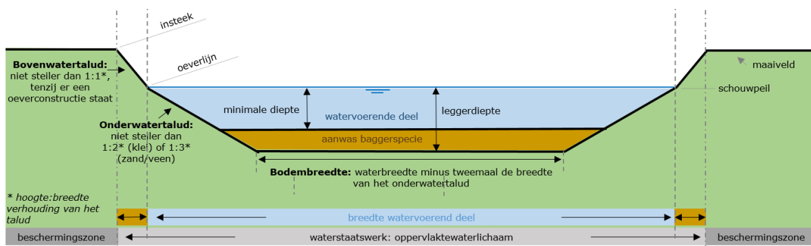
Figuur 29: Voorbeeldsituatie 2: leggerprofiel watervoerend deel van een 'brede watergang'. Bij brede watergangen neemt de diepte niet meer rechtlijnig toe met de breedte; het omslagpunt ligt bij een onderwatertalud met een helling van 1:5.
