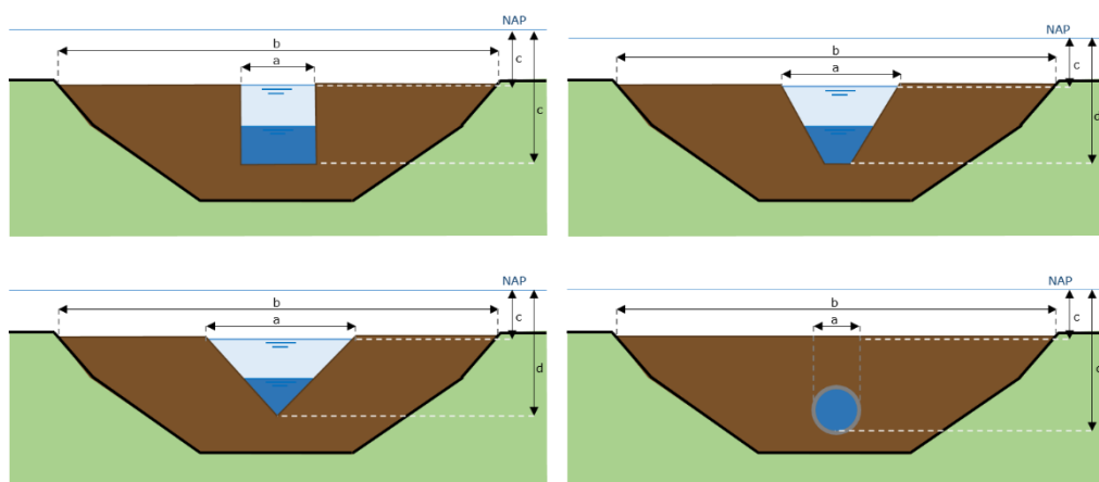
Figuur 38: Schematische weergave leggerprofiel (dwarsprofiel) van een stuw. Afmetingen: doorstroombreedte (a), kruinbreedte (b), hoogste doorstroomhoogte (c), laagste doorstroomhoogte (d). Deze afmetingen staan op het informatiescherm van de stuw op de leggerkaart. De hoogte wordt weergegeven ten opzichte van N.A.P.
