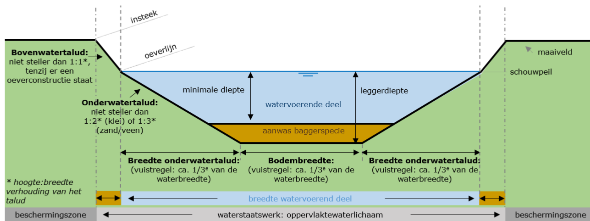
Figuur 28: Voorbeeldsituatie 1: leggerprofiel watervoerend deel van een 'gemiddelde watergang'. Deze situatie kan van toepassing zijn in situaties waarbij het onderwatertalud gelijk aan of flauwer is dan 1:2 (klei) of 1:3 (zand/veen), maar steiler dan 1:5.
