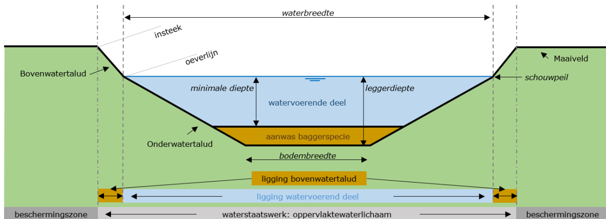
Figuur 23: Schematische weergave standaard trapeziumvormig leggerprofiel van een oppervlaktewaterlichaam. Het oppervlaktewaterlichaam bestaat uit het watervoerend deel en het bovenwatertalud. Het standaard leggerprofiel van het watervoerend deel heeft een trapezium vorm. De zone van het bovenwatertalud loopt van de oeverlijn tot de insteek. De beschermingszone grenst aan het oppervlaktewaterlichaam. De figuur toont de samenhang tussen de verschillende begrippen die met een oppervlaktewaterlichaam en de bijbehorende beschermingszone te maken hebben.
