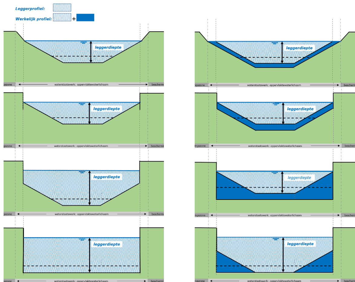
Figuur 4: Voorbeeldsituaties: relatie werkelijk aanwezig (dwars)profiel in relatie tot het leggerprofiel van het watervoerend deel van een oppervlaktewaterlichaam. Afbeeldingen links: het werkelijk aanwezige profiel is gelijk aan het leggerprofiel; Afbeeldingen rechts: het werkelijk aanwezige profiel is groter dan het leggerprofiel.
