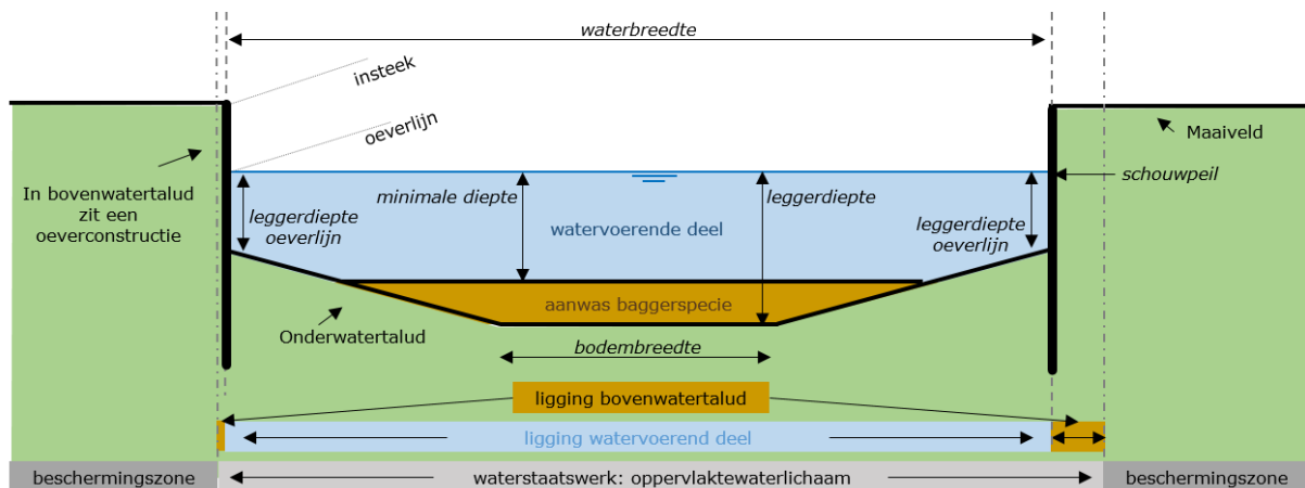
Figuur 27: Schematische weergave bak-vorm leggerprofiel van het watervoerend deel. Een leggerdiepte aan de oeverlijn geeft aan dat het trapezium leggerprofiel niet van toepassing is. Let op: de werkelijke diepte van het watervoerend deel kan dieper zijn dan het leggerprofiel.
