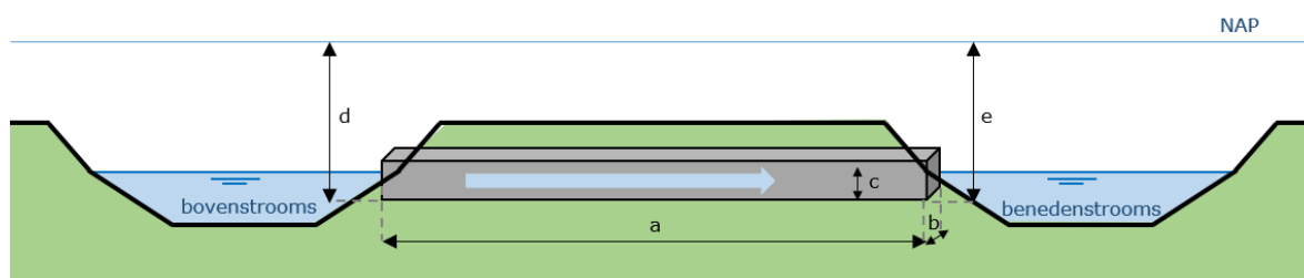
Figuur 37: Schematische weergave leggerprofiel van een duiker. Afmetingen: lengte (a), breedte opening (b), hoogte opening (c), hoogte binnen onderkant bovenstrooms (d), hoogte binnen onderkant benedenstrooms (e). Deze afmetingen staan op het informatiescherm van de duiker op de leggerkaart. De hoogte wordt weergegeven ten opzichte van N.A.P.
