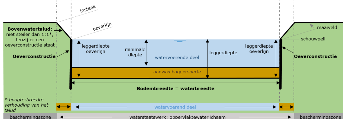
Figuur 35: Voorbeeldsituatie 8: leggerprofiel watervoerend deel, type: bak-profiel. Deze situatie is van toepassing als er vanuit een waterhuishoudkundig oogpunt een bak-profiel vereist is. Deze situatie is van toepassing als er op de leggerkaart aan twee zijden van de watergang een leggerdiepte op de oeverlijn staat aangegeven en deze gelijk is aan de leggerdiepte (in het midden van de watergang).
