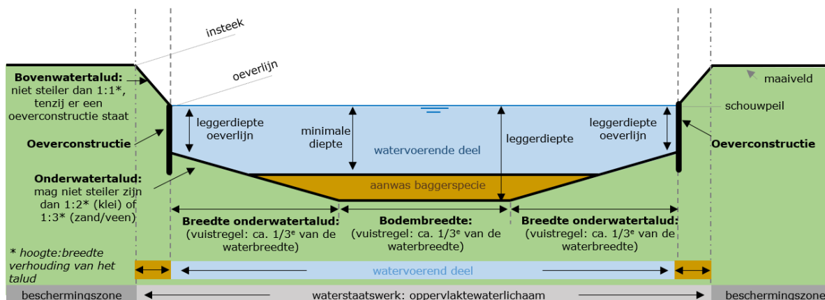
Figuur 33: Voorbeeldsituatie 6: leggerprofiel watervoerend deel, type: U-profiel. Deze situatie is van toepassing als er vanuit een waterhuishoudkundig oogpunt een U-profiel vereist is. Op de leggerkaart staan dan een leggerdiepte op de oeverlijn aan twee zijden van de watergang staat aangegeven.
