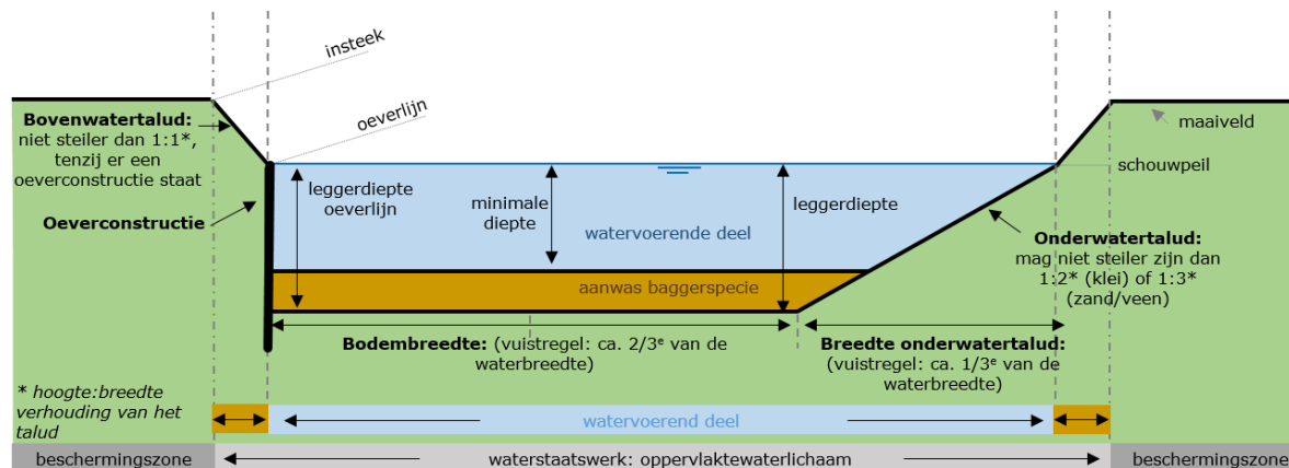
Figuur 34: Voorbeeldsituatie 7: leggerprofiel watervoerend deel, type: half-bak-profiel. Deze situatie is van toepassing als er vanuit een waterhuishoudkundig oogpunt een half-bak-profiel vereist is. Deze situatie is van toepassing als er op de leggerkaart aan één zijde van de watergang een leggerdiepte op de oeverlijn staat aangegeven en deze gelijk is aan de leggerdiepte (in het midden van de watergang).
