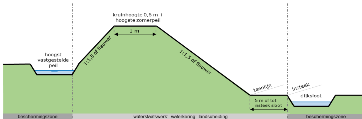
Figuur 21: Voorbeeld van een locatie specifiek leggerprofiel voor de landscheiding. Dit leggerprofiel is bepaald aan de hand van Artikel 2.6 Ligging en afmeting van landscheidingen en bijbehorende beschermingszone in de legbertekst
