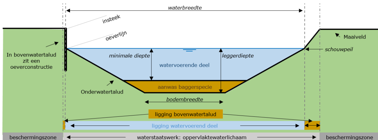
Figuur 26: Schematische weergave leggerprofiel van een oppervlaktewaterlichaam met oeverconstructie. De aanwezigheid van een oeverconstructie verandert het normatieve leggerprofiel van het watervoerend deel niet. Let op: de werkelijke afmetingen van het watervoerend deel kunnen breder en dieper zijn dan het leggerprofiel.
