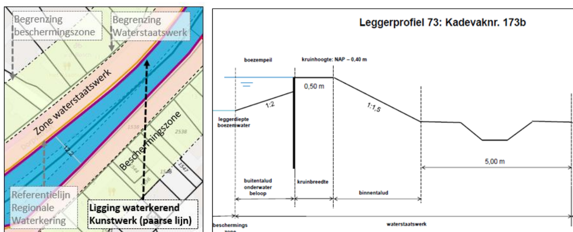
Figuur 17: Voorbeeld weergave: Ligging regionale waterkering (met waterkerend kunstwerk) op leggerkaart en bijbehorend locatie specifiek leggerprofiel
