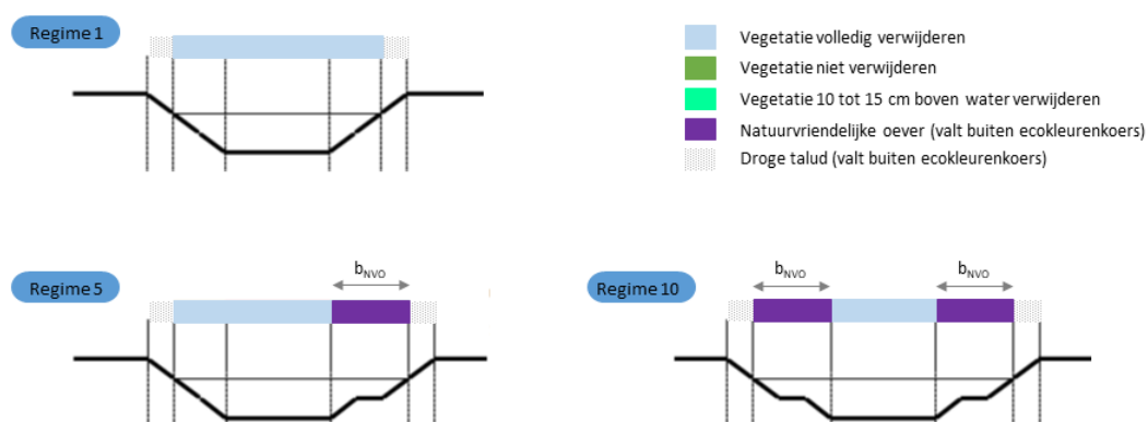
Afbeelding 2 Dwarsdoorsnede watergang met te voeren onderhoudsregime ecokleur blauw. (er komen nieuwe illustraties)
