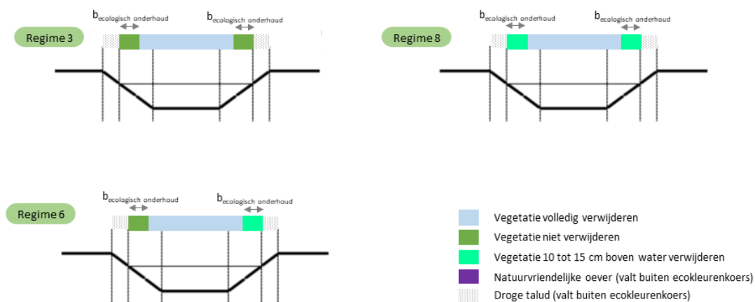
Afbeelding 4 Dwarsdoorsnede met de te voeren maairegime ecokleur groen. (er komen nieuwe illustraties)
