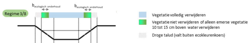
Afbeelding 9 Visualisatie maairegime groene secundaire watergangen (er komen nieuwe illustraties)
