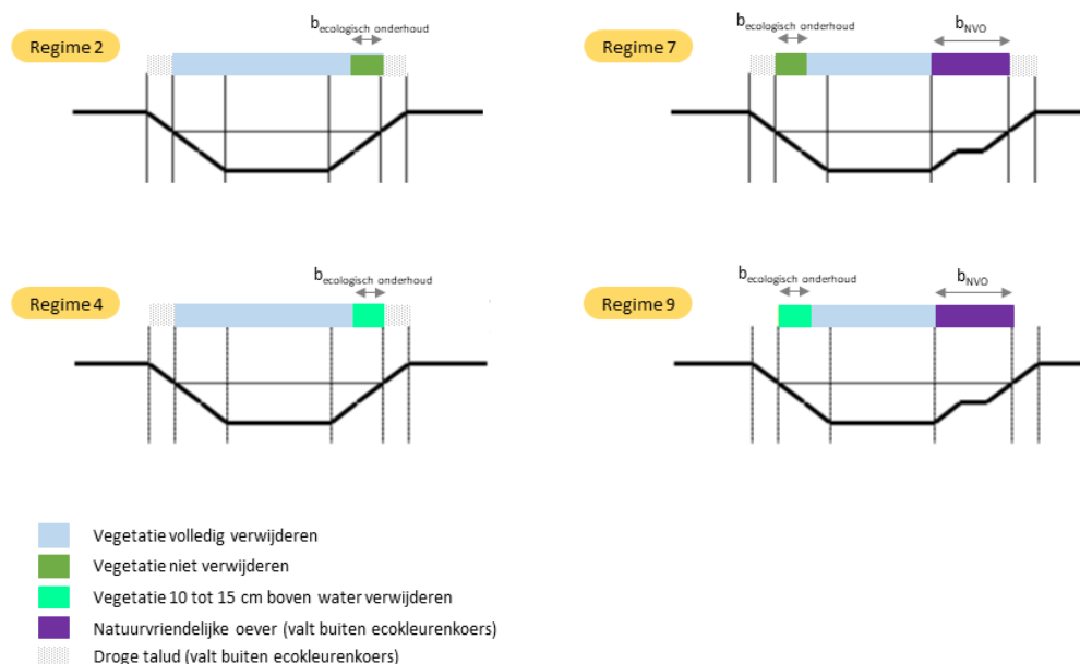
Afbeelding 3 Dwarsdoorsnede met de te voeren maairegime ecokleur geel. (er komen nieuwe illustraties)
