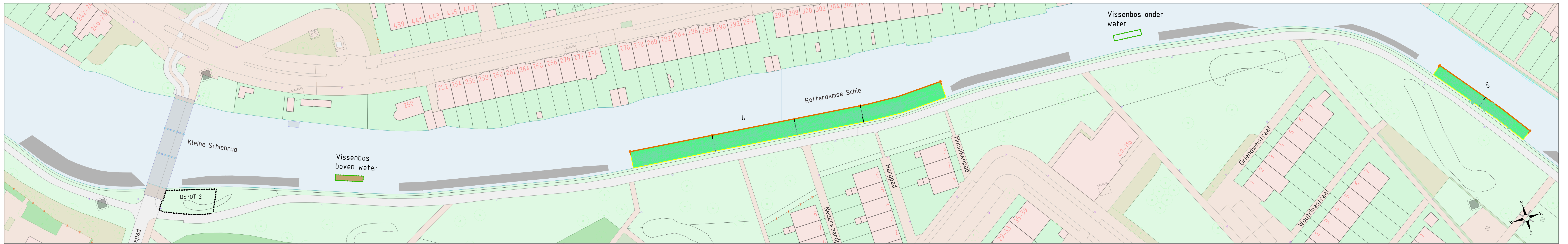
Situatie midden SCHAAL 1 : 500
